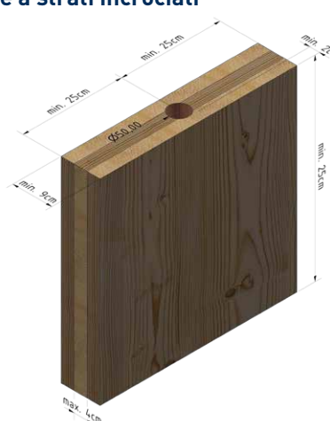
Movimentazione verticale di legno lamellare a strati incrociati
