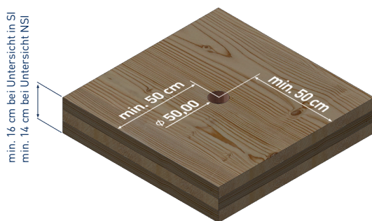
Horizontale Manipulation von BSP
