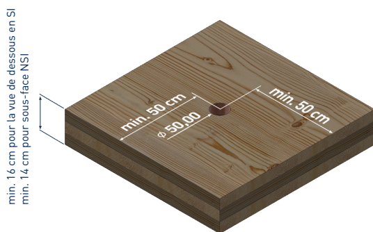
Manipulation horizontale de bois contrecollé
